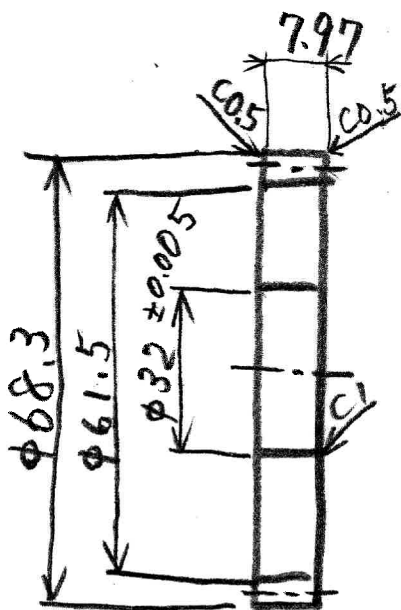
遊星歯車
