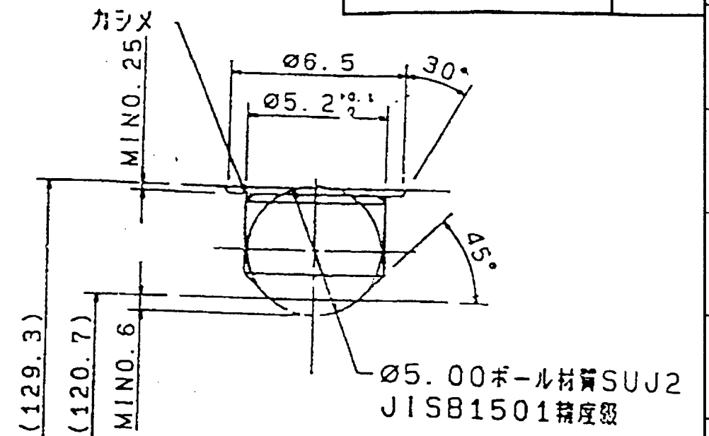
ボール穴部詳細 (S=5/1)
